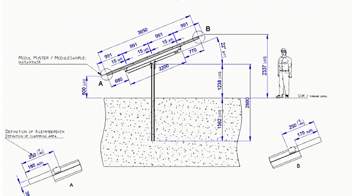
Modultischkonstruktion, Option 1 ohne Maßstab
